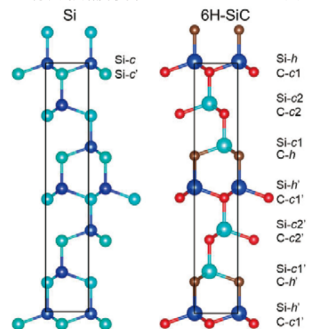
シリコン(Si)と6H型炭化ケイ素(6H-SiC)の結晶構造。シリコンは一つの結晶サイトしか存在しないが、6H型炭化ケイ素は6つの結晶サイトが存在する。
